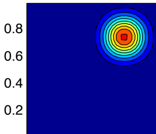
3-DST Sweby \mu=\mu(c)
